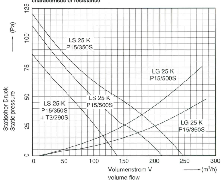
Leistungsdiagramm mit Widerstandskennlinie
